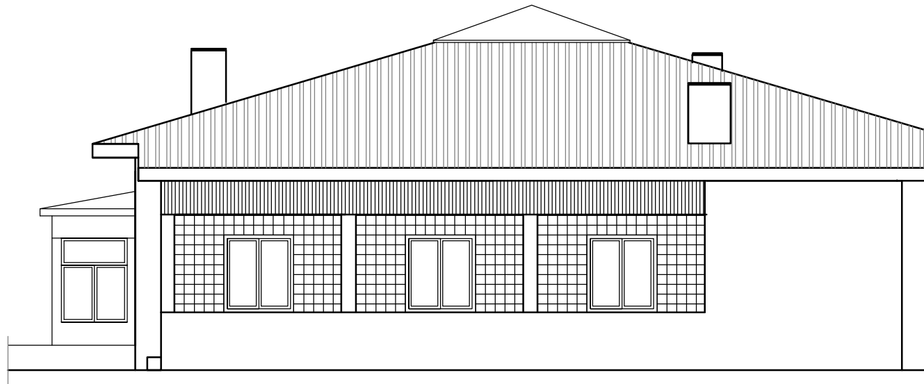
ALZADO ESTE
