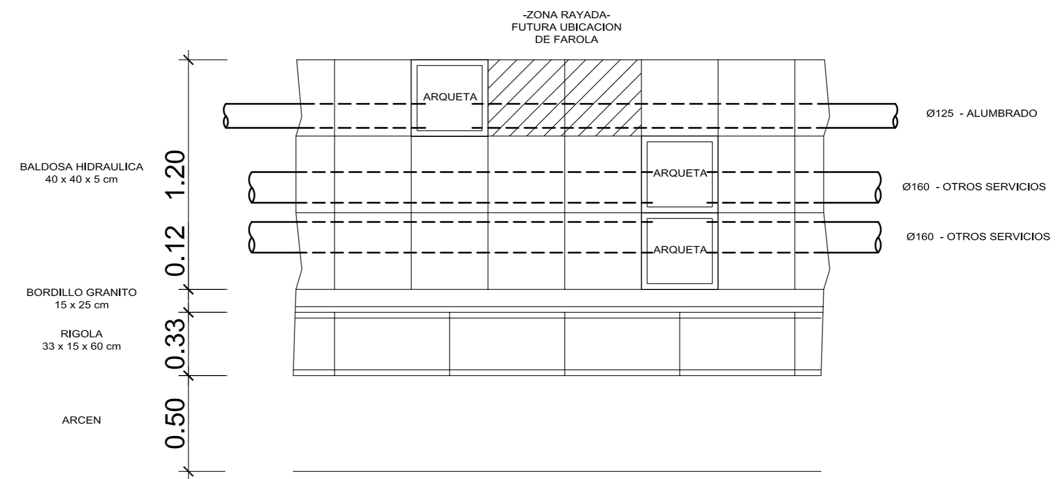
DETALLE DE PLANTA DE ACERA ESCALA 1/20
