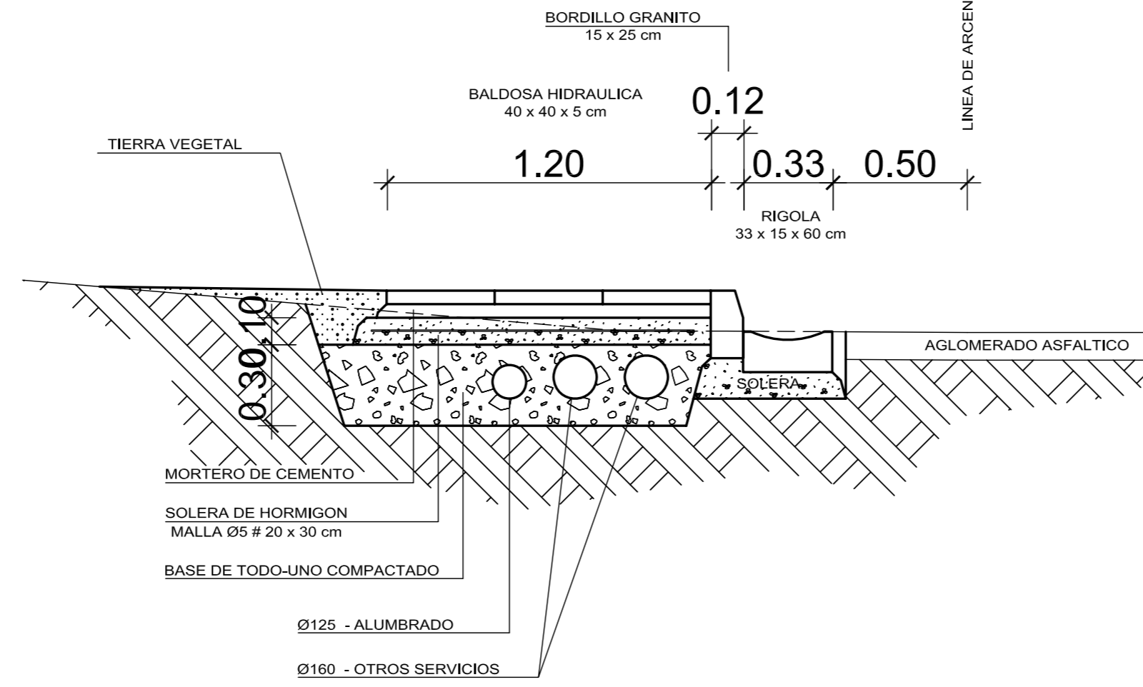
DETALLE DE SECCIONES ESCALA 1/20
