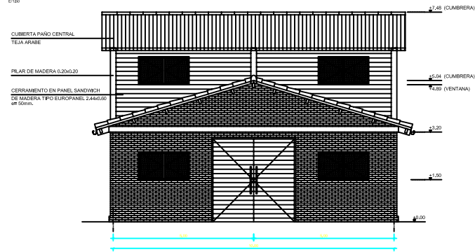
ALZADOS ESTE-OESTE E108
