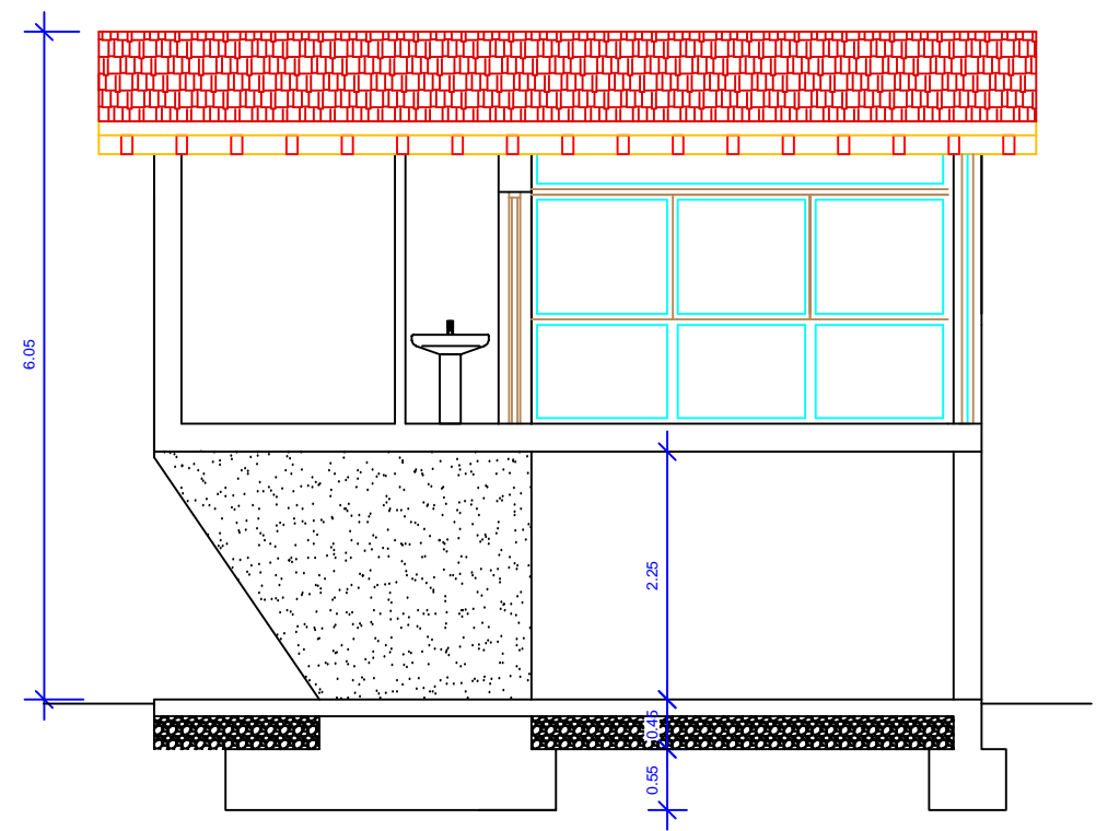
SECCION A-A'
