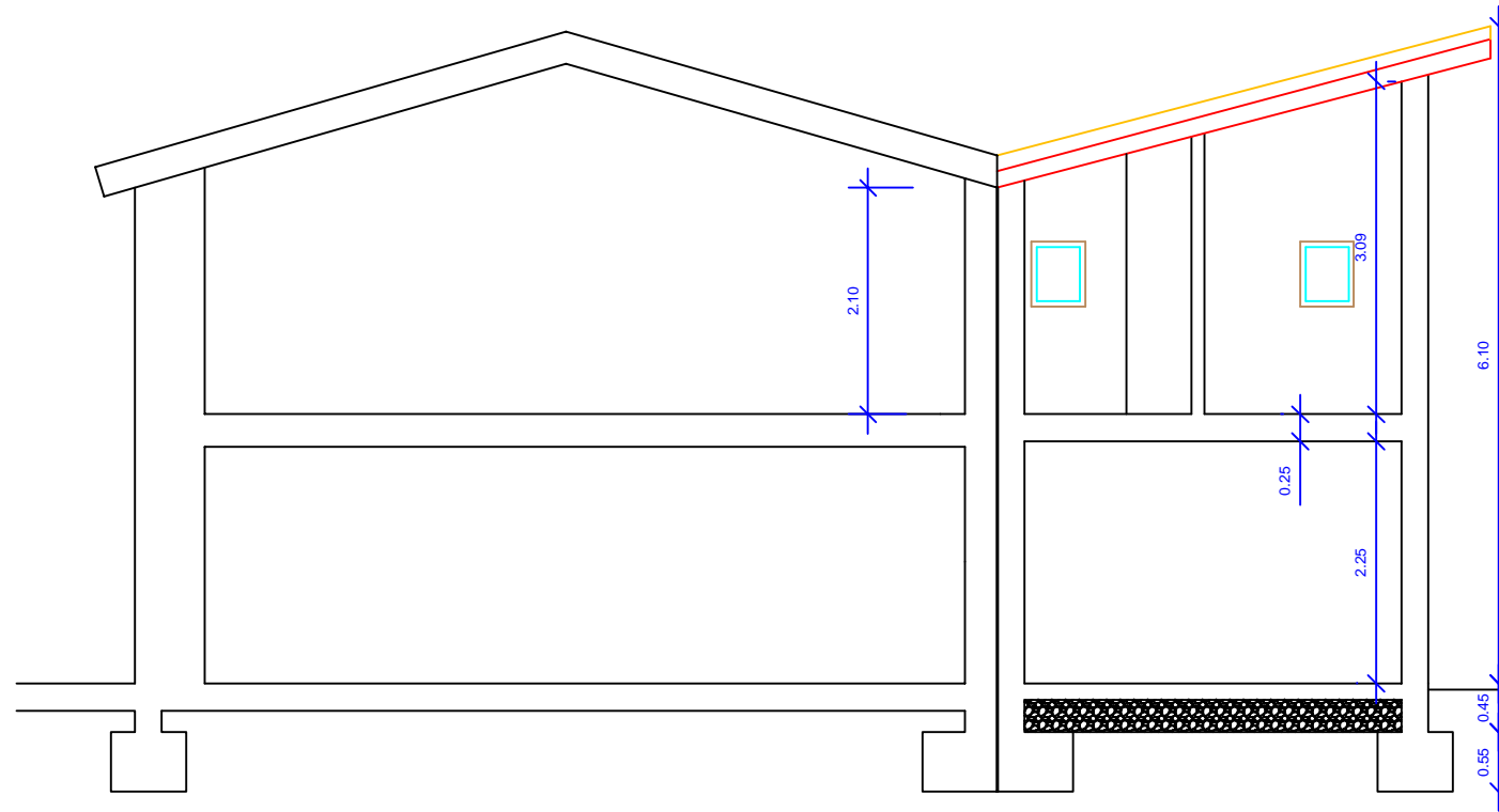
SECCION B-B'
